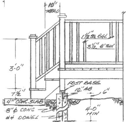
STAIR DETAIL SCALE: 3/8" = 1'-0"
